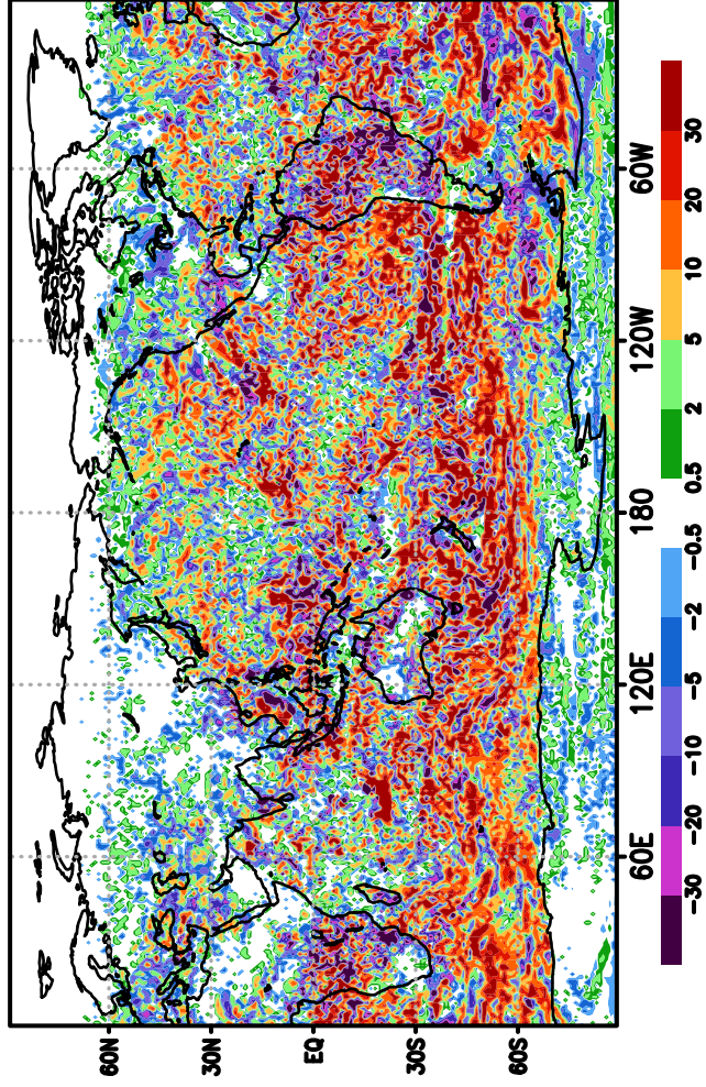
fv3gradr2 dswrfsfc (3.138,2.412)
